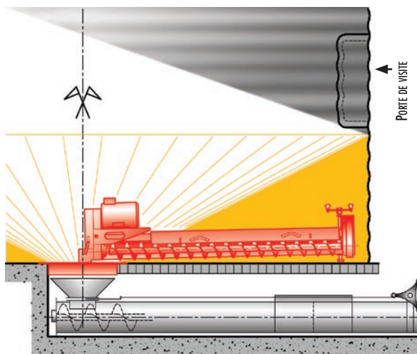
Exemple d'implantation avec reprise par vis horizontale.
