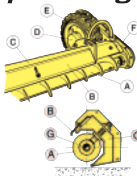
Vidange du cône résiduel Residual grain discharge
